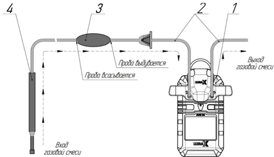
Рисунок Г.2 – Схема соединения ручного насоса и газоанализатора 1- Газоанализатор AVIS X4 с калибровочной насадкой; 2 - Трубка силиконовая 6х4 – 2 шт. по 1,5 м; 3 - Мех резиновый; 4 - Зонд телескопический.
