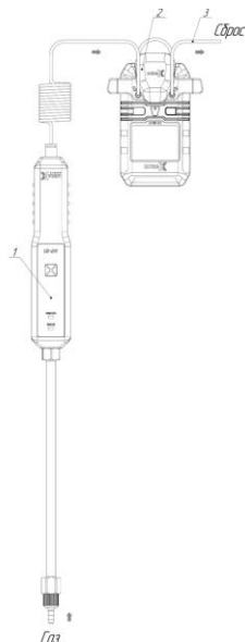
Рисунок Д.2 – Схема соединения моторизированного насоса и газоанализатора 1– Насос; 2 – Калибровочная насадка; 3– Сброс
