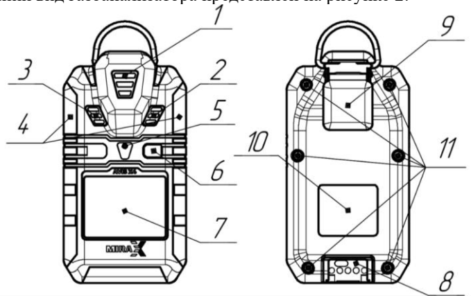
Рисунок 2 – Внешний вид газоанализатора
