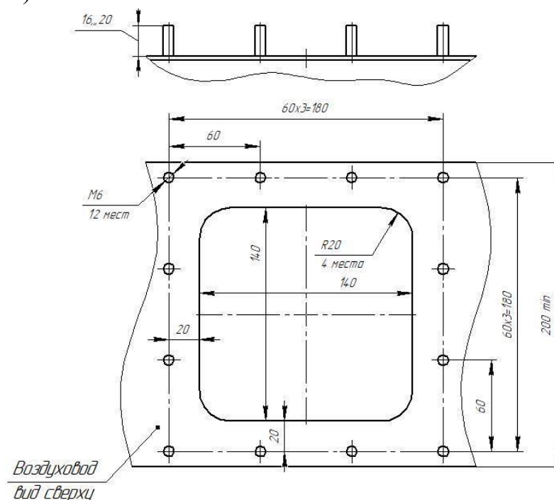
Рисунок 30 – Место для установки комплекта
