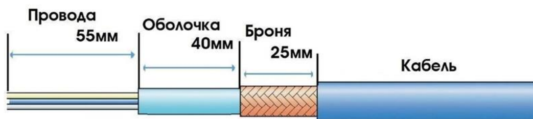
Рисунок 25 – Подготовка кабеля с бронезащитой
