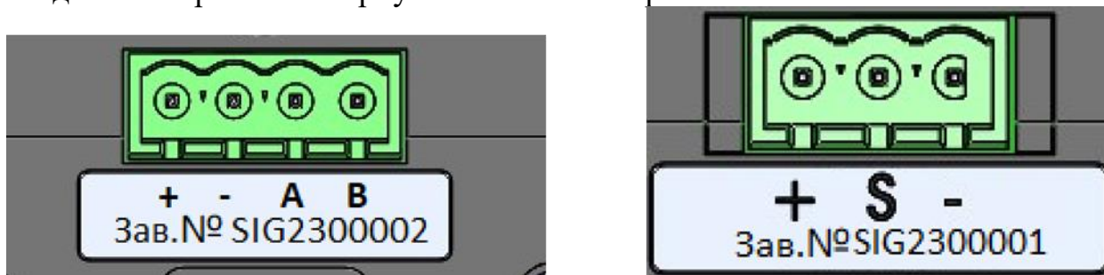
Рисунок 32 – Схема подключения газоанализатора SIGNAL
