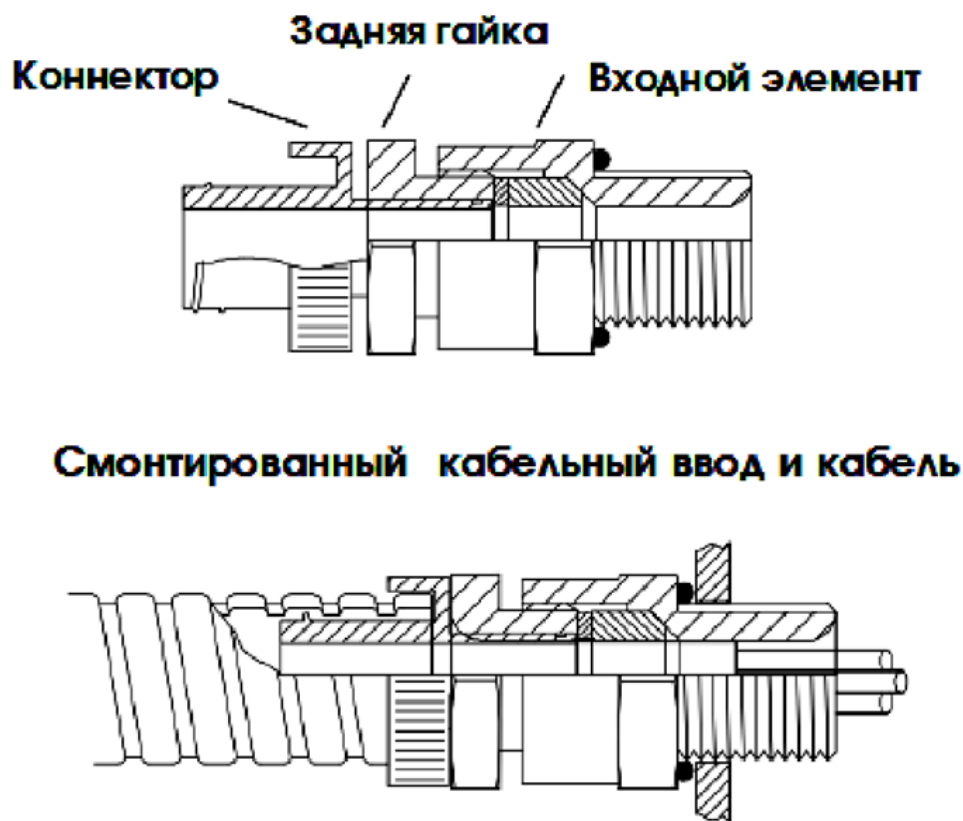
Рисунок 22 - Кабельный ввод
